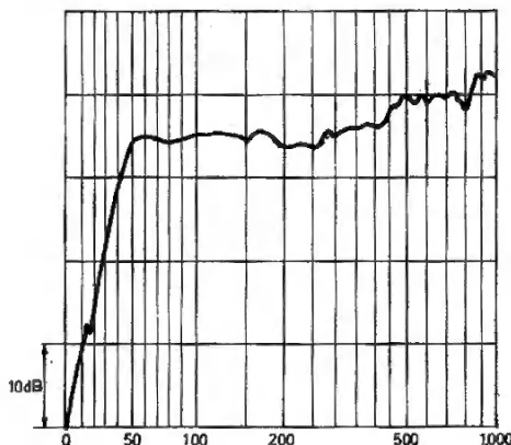
Frequentiekaracteristiek van de „Bombardon” (AD 1255/W8)
